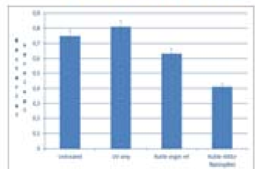
TiO 2 Flat rutile vs nanospikes
